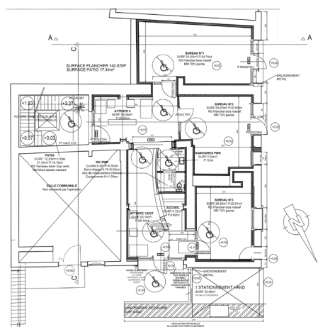
► Plan du rez-de-chaussée - Permis déposé.
