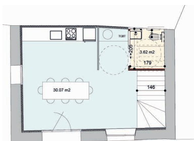
► Plan du RDC.
