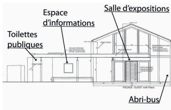
► Esquisse du projet.
