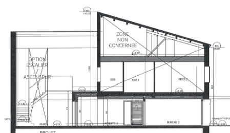
► Coupe du bâtiment vue de l'Église.
